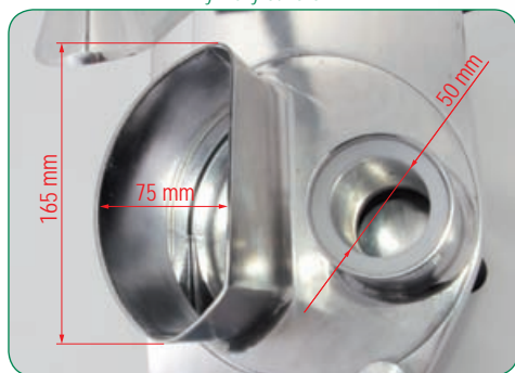
wymiary otworów
